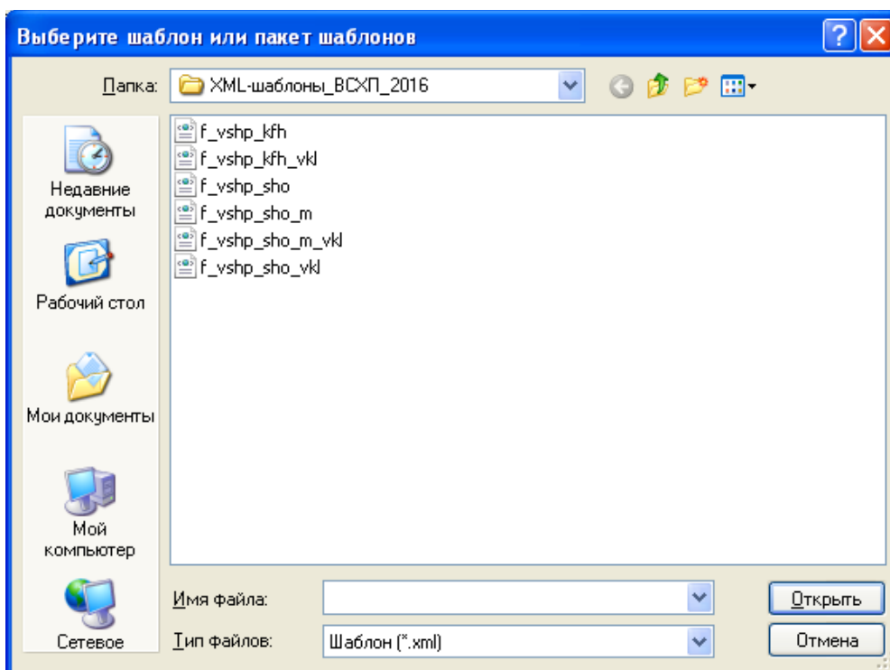
Рисунок 10 – Выбор XML-Шаблона
